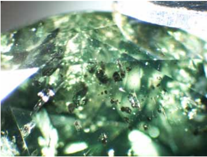
Рисунок 2. Графітоподібні включення і тріщини в діаманті. Збільшення 36 x
