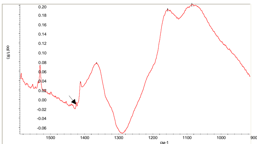
Рисунок 5. Облагороджені алмази змішаного типу Ib+IaA (пік 1282 \text{cm}^{-1} , 1344 \text{cm}^{-1} ) фіолетового кольору
