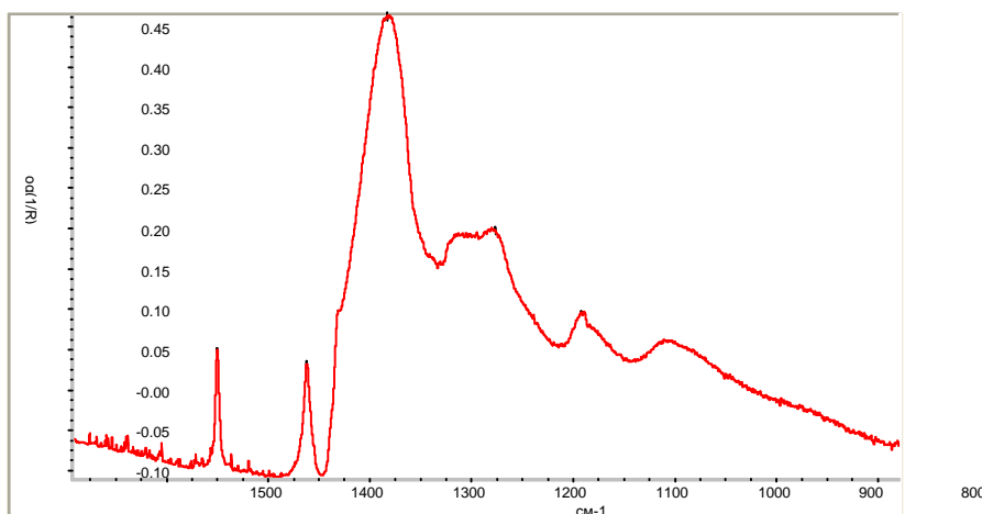
Рисунок 3. Облагорожені алмази типу IaAB (пік 1282\text{ cm}^{-1} , 1175\text{ cm}^{-1} ) жовто-зеленого кольору
