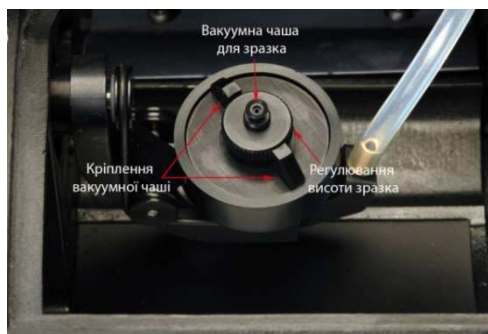
Рисунок 6. Зовнішній вигляд приладу «Diamond View» та його внутрішня будова
