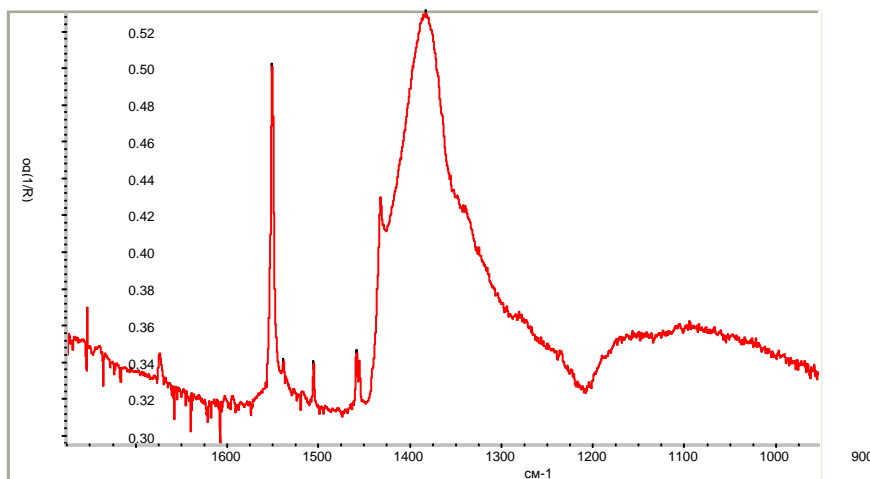
Рисунок 2. Облагорожені алмази типу IaA (пік 1282\text{ cm}^{-1} ) жовто-оранжевого кольору
