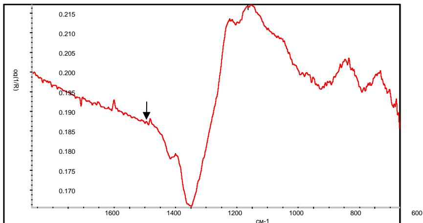
Рисунок 4. Облагороджені алмази типу Ib (пік 1344 \text{cm}^{-1} ) фіолетового кольору
