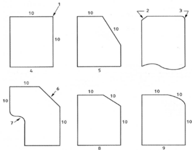
Рисунок 2. Типи бордюрів з декоративного камення в перетині відповідно до ДСТУ EN 1343:2007
