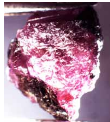
Рисунок 1. Загальний вигляд олександриту при денному освітленні (ліворуч) і при штучному освітленні (праворуч), зб. 20
